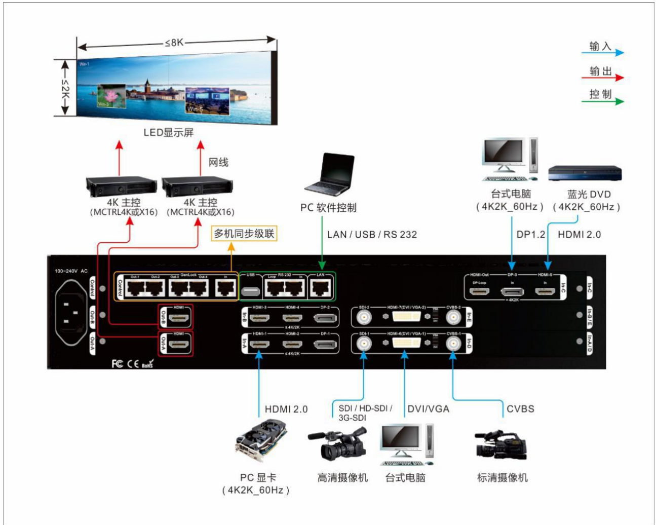
硬件连接图-配置模式 1 (CfgM1)
