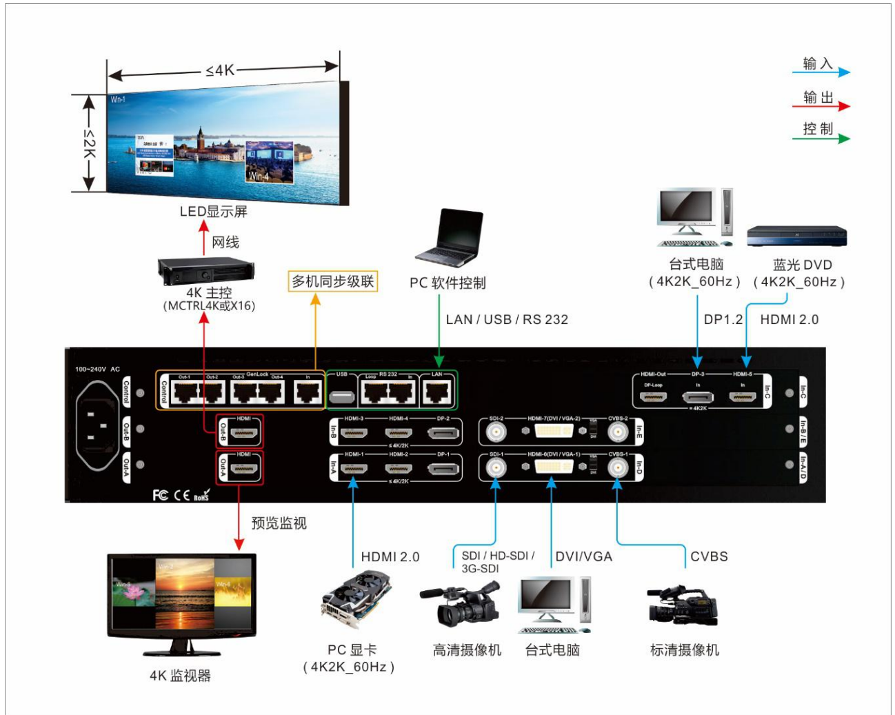
硬件连接图-配置模式 0 (CfgM0)
