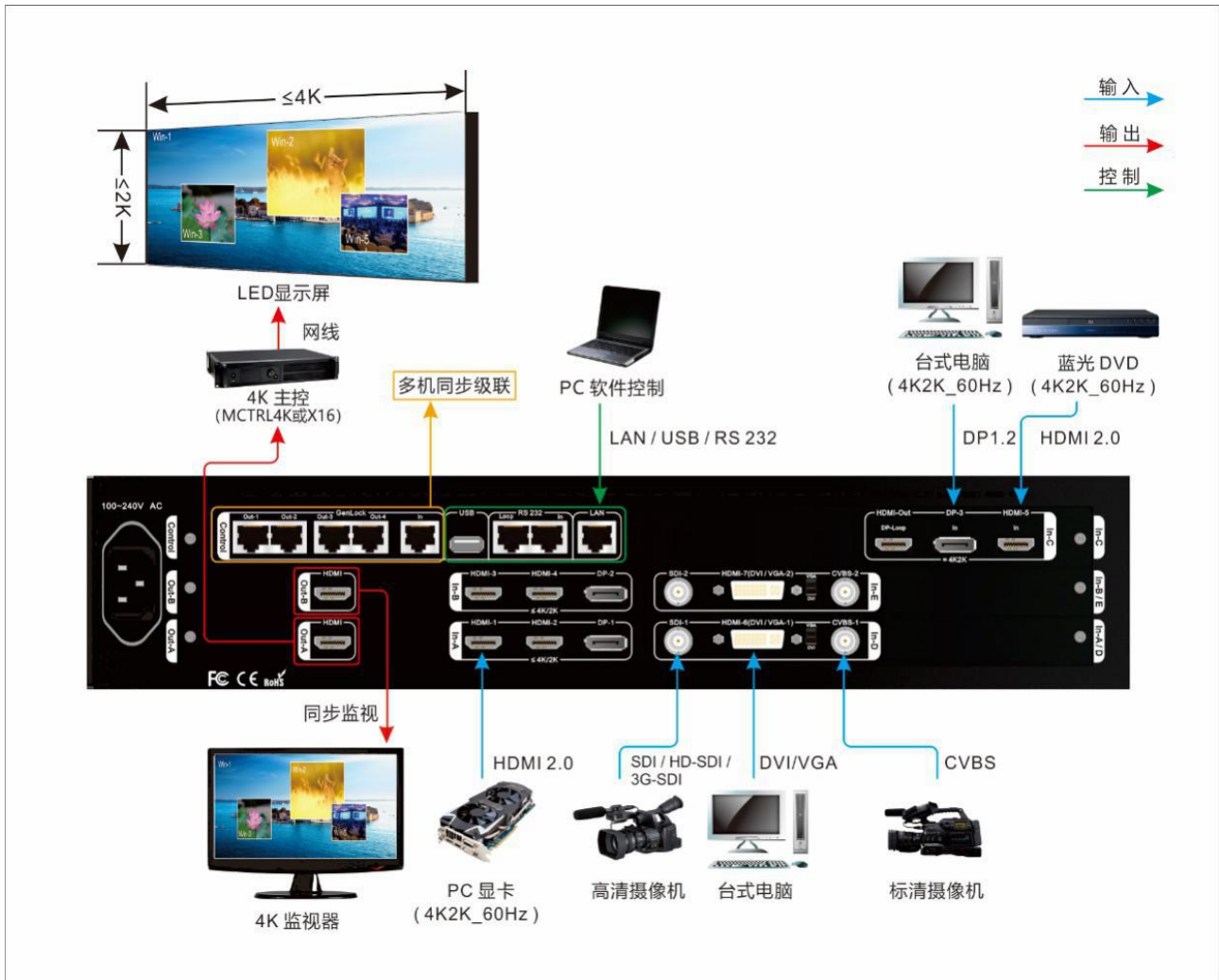
硬件连接图-配置模式 2 (CfgM2)
